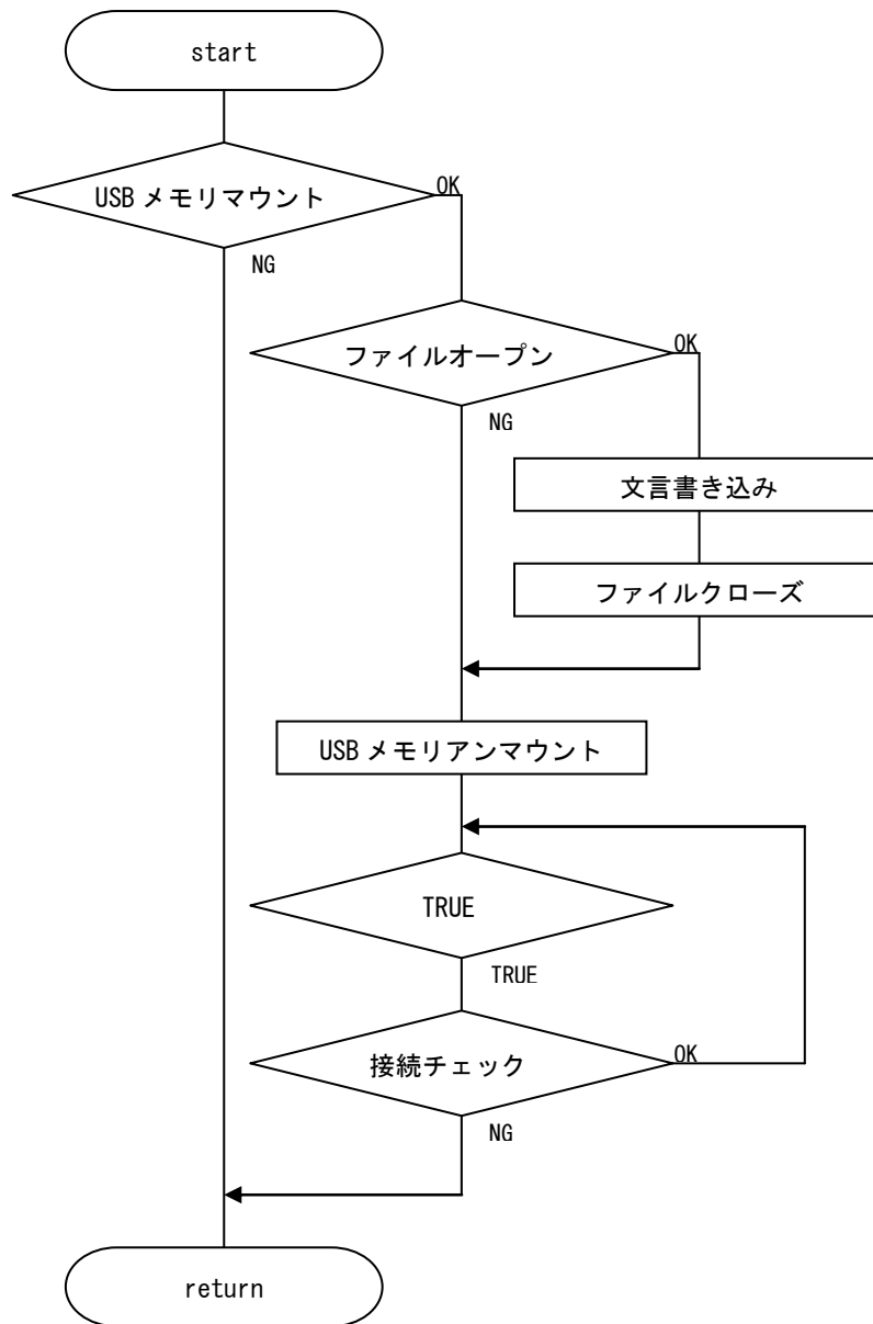
図 3.3 アプリケーション処理フロー
