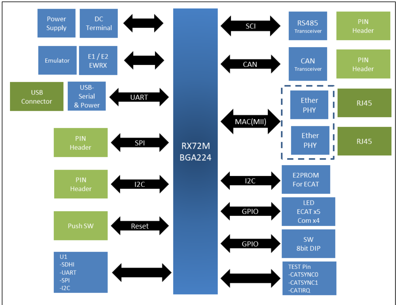
図 1-1 全体ブロック図
