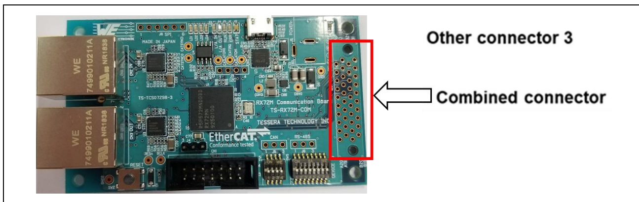
図 3-11 集合コネクタ
