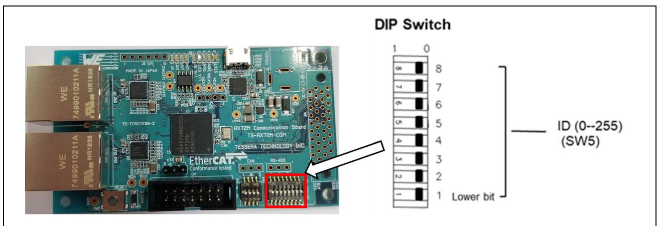
図 3-7 ディップスイッチ
