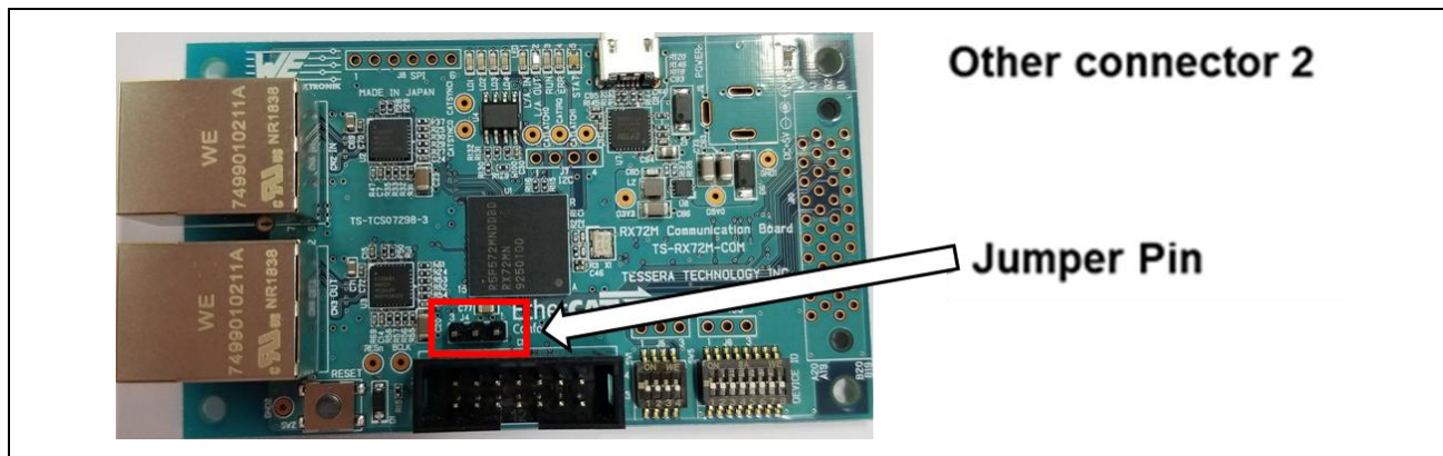
図 3-10 ジャンパーピン
