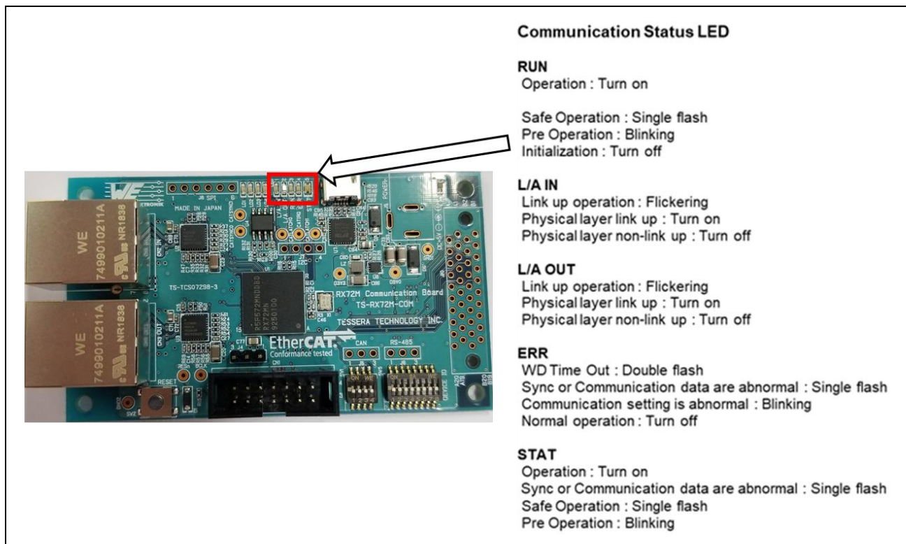
図 3-4 EtherCAT 通信ステータス LED
