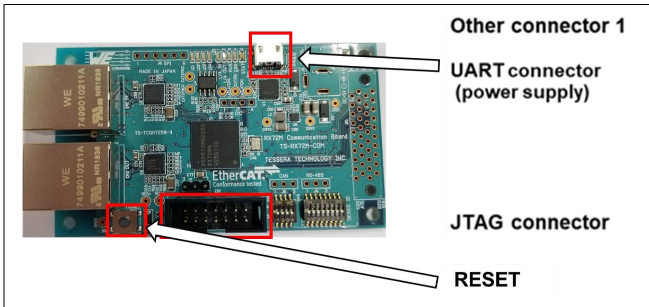
図 3-8 基板スイッチ
