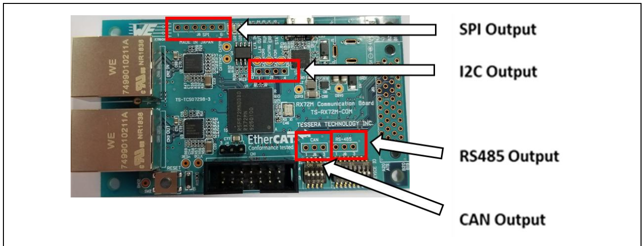
図 3-3 電源、I/O コネクタ
