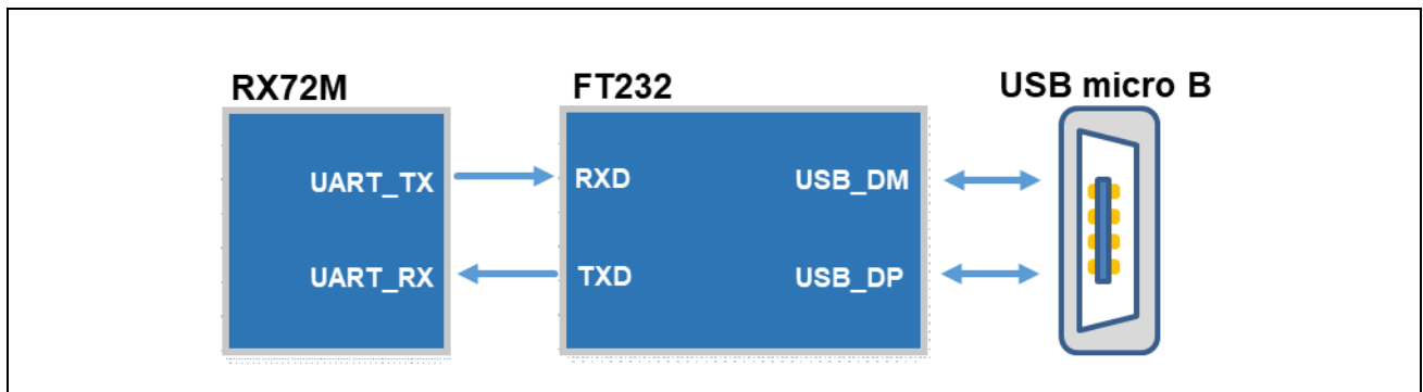
図 3-9 UART
