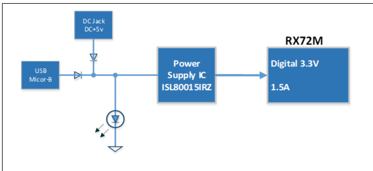
図 3-6 外部電源供給図
