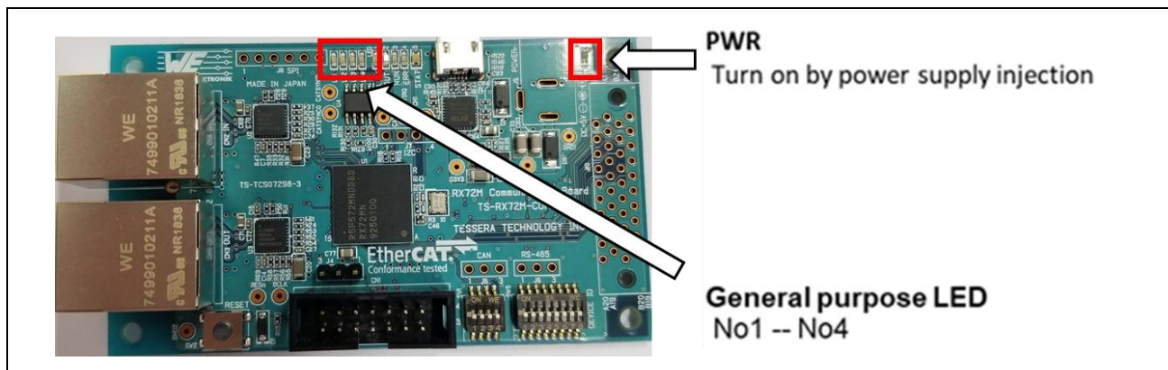
図 3-5 電源・汎用 LED
