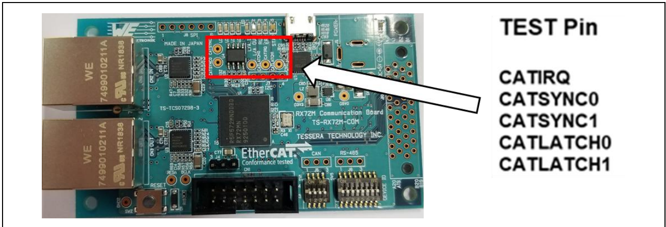
図 3-5 テストピン
