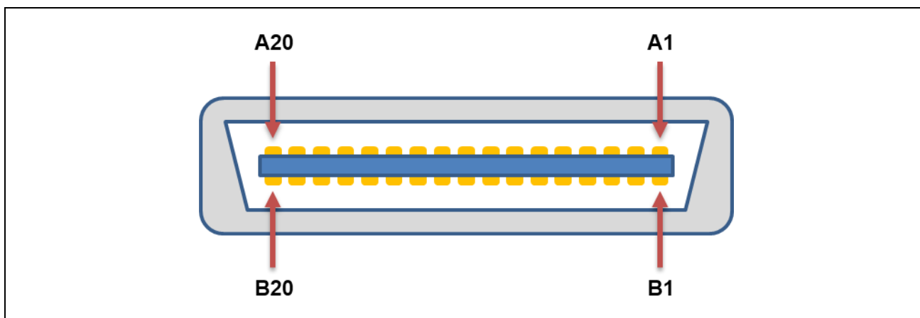
図 3-4 集合コネクタピン配置
